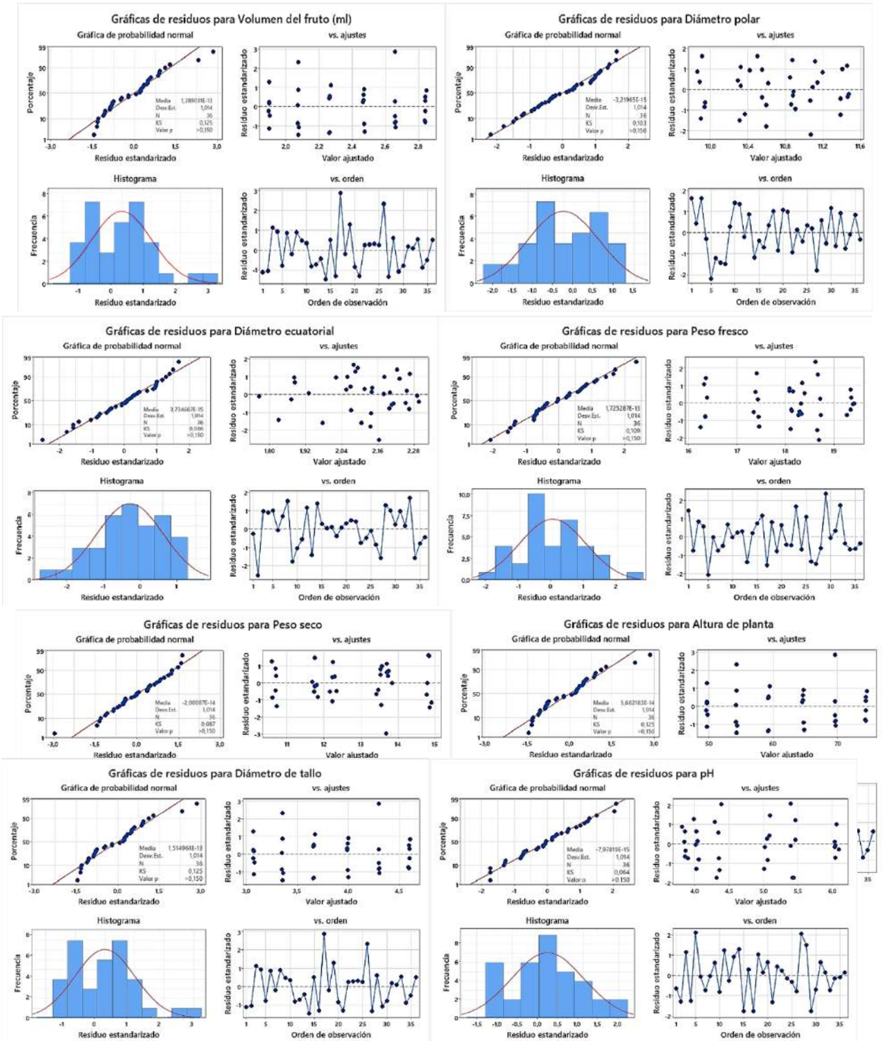
Figura 1. Gráficas de los residuos donde se muestran las gráficas de probabilidad normal (Q-Q plot); graficas de residuos estandarizados vs. ajustes (homocedasticidad); histogramas de los residuos y; gráficas de los residuos estandarizados vs orden de observación (Independencia) para cada variable respuesta.
