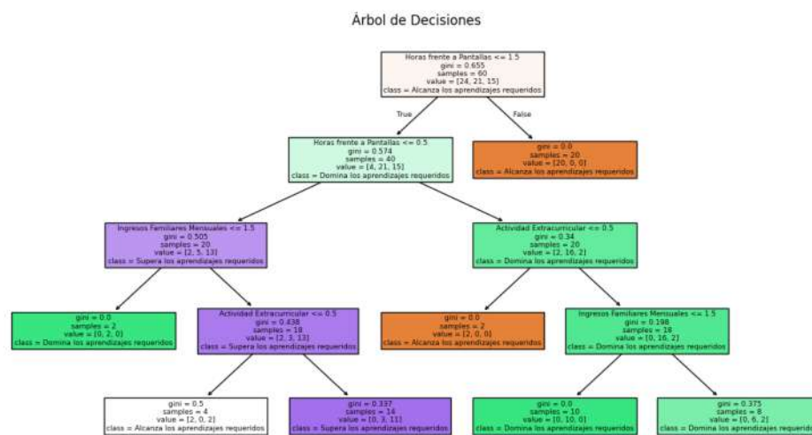
Figura 2. Representación gráfica del árbol de decisión utilizado en el estudio.
