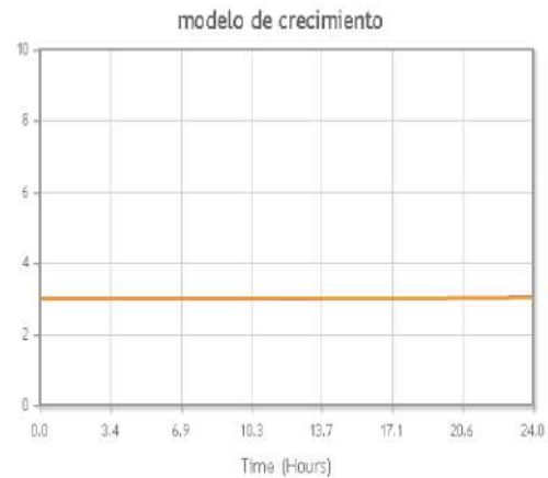
Figura 5. Curva de crecimiento E. coli y S. aureus (día 1) T3.
