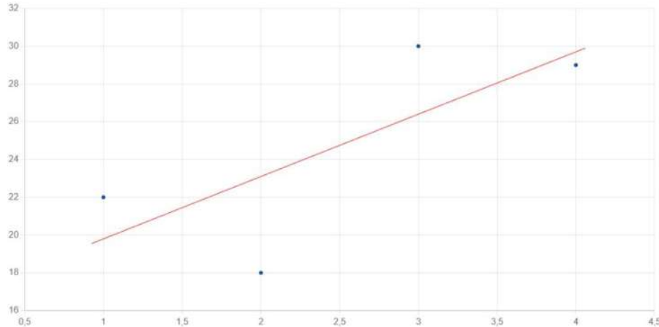
Figura 1. Correlación de Pearson.
